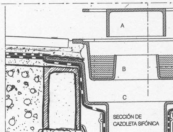
PERSPECTIVA SECCIONADA DE LA CAZOLETA SIFÓNICA
