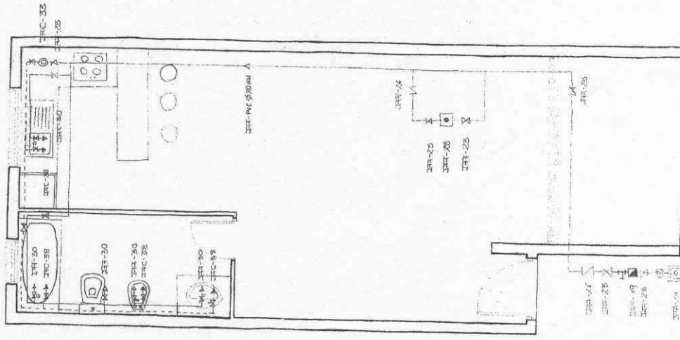
PLANTA DE FONTANERÍA: I.F.F.:
